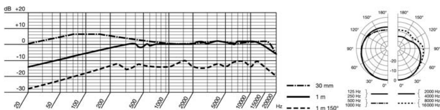
Frequenzgang und Polardiagramm HSC 171, HSC 271
